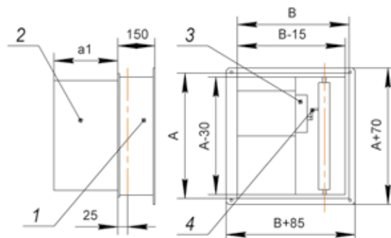
Сигмавент-120(180)-НЗ(С)-АхВх150-...
