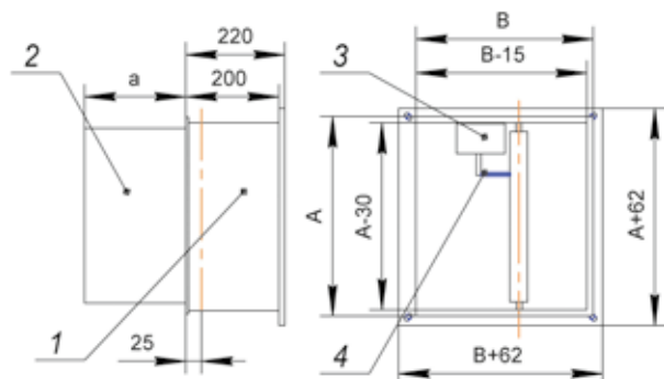
Сигмавент-120(180)-НЗ(С)-АхВ-...
